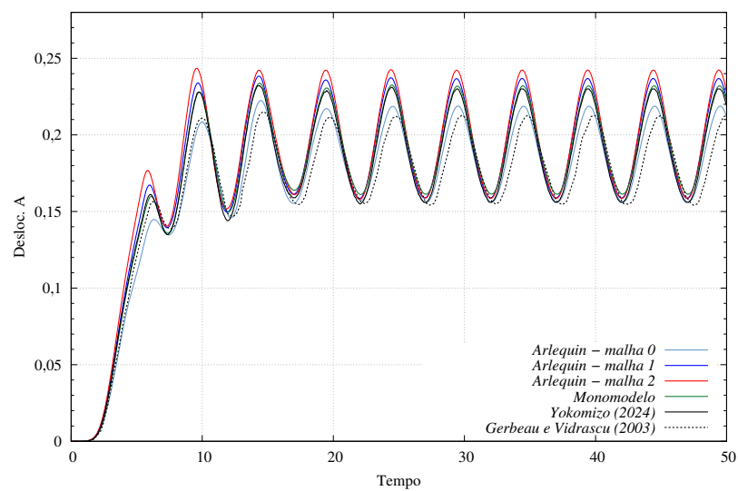
Figura 77 – Cavity com fundo flexível 2D: deslocamento do ponto A
