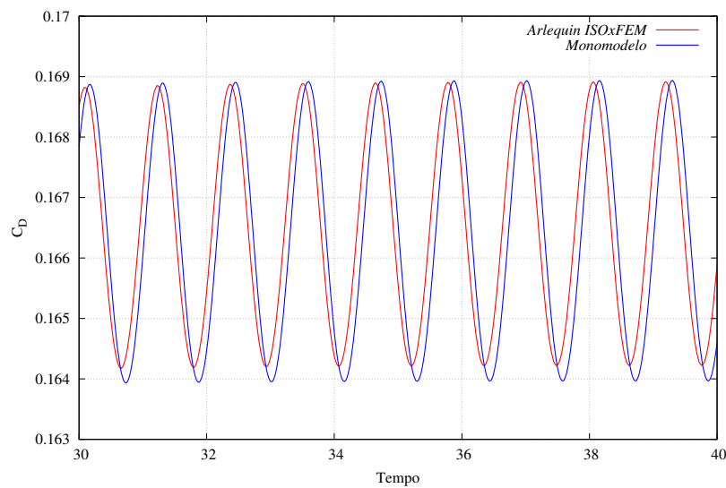
Figura 64 – Aerofólio: coeficiente de arrasto
