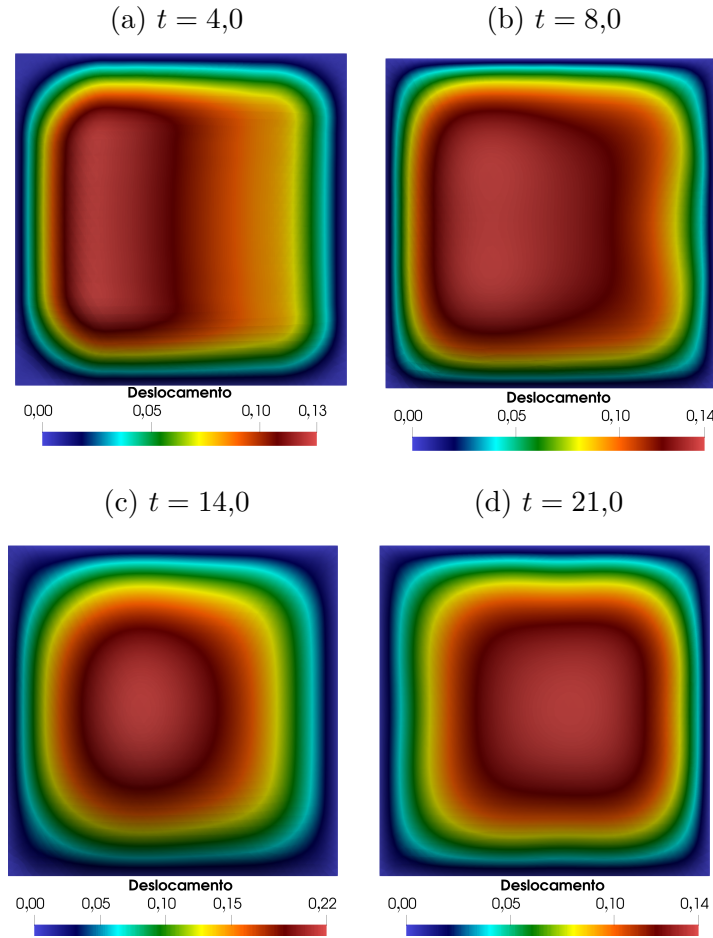
Figura 85 – Casca: campo de deslocamento
