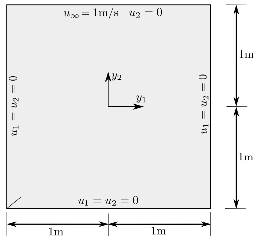
Figura 51 – Cavidade: geometria e condições de contorno
