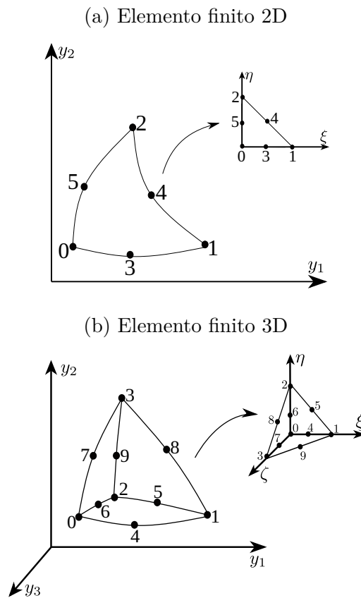
Figura 6 – Elementos finitos: representação espacial e paramétrica
