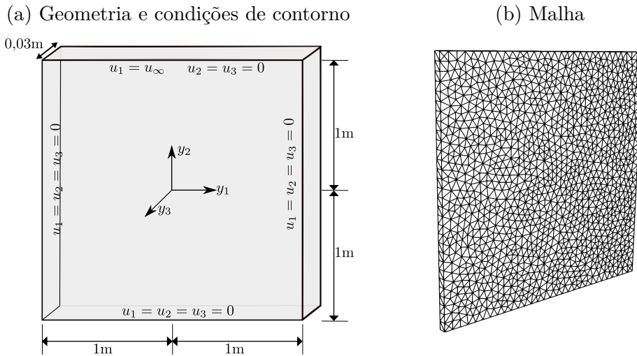
Figura 11 – Cavidade: geometria, condições de contorno e malha
