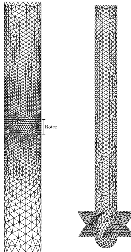
Figura 94 – Turbina monomodelo: malhas
