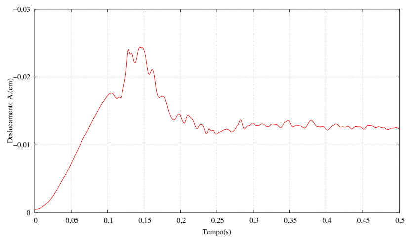
Figura 95 – Turbina monomodelo: deslocamento no ponto A
