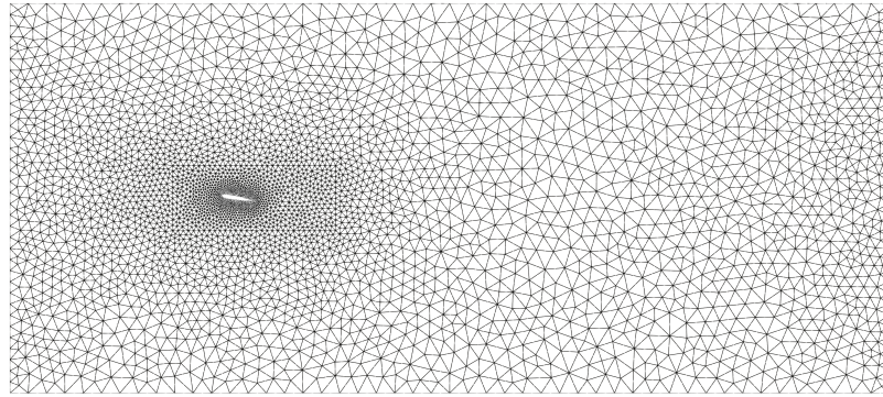
Figura 62 – Aerofólio: malha monomodelo (MEF)
