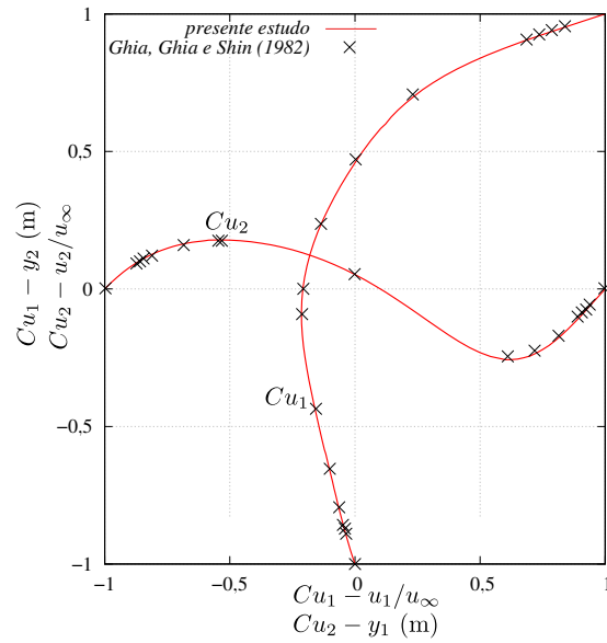
Figura 54 – Cavity: perfil de velocidade adimensionalizado
