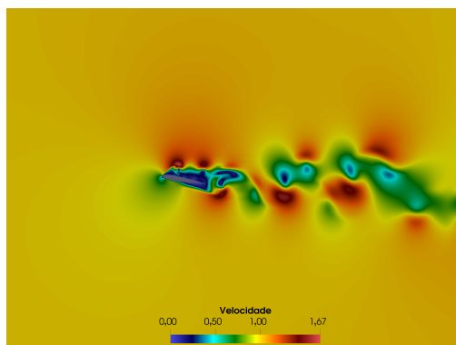
Figura 71 – Aerofólio Mov.: campo de velocidade
