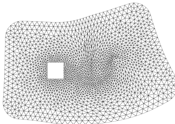
Figura 90 – PAINEL flexível: deformada da malha em nT
