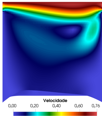
Figura 83 – Cavity com fundo flexível 3D: campo de velocidade
