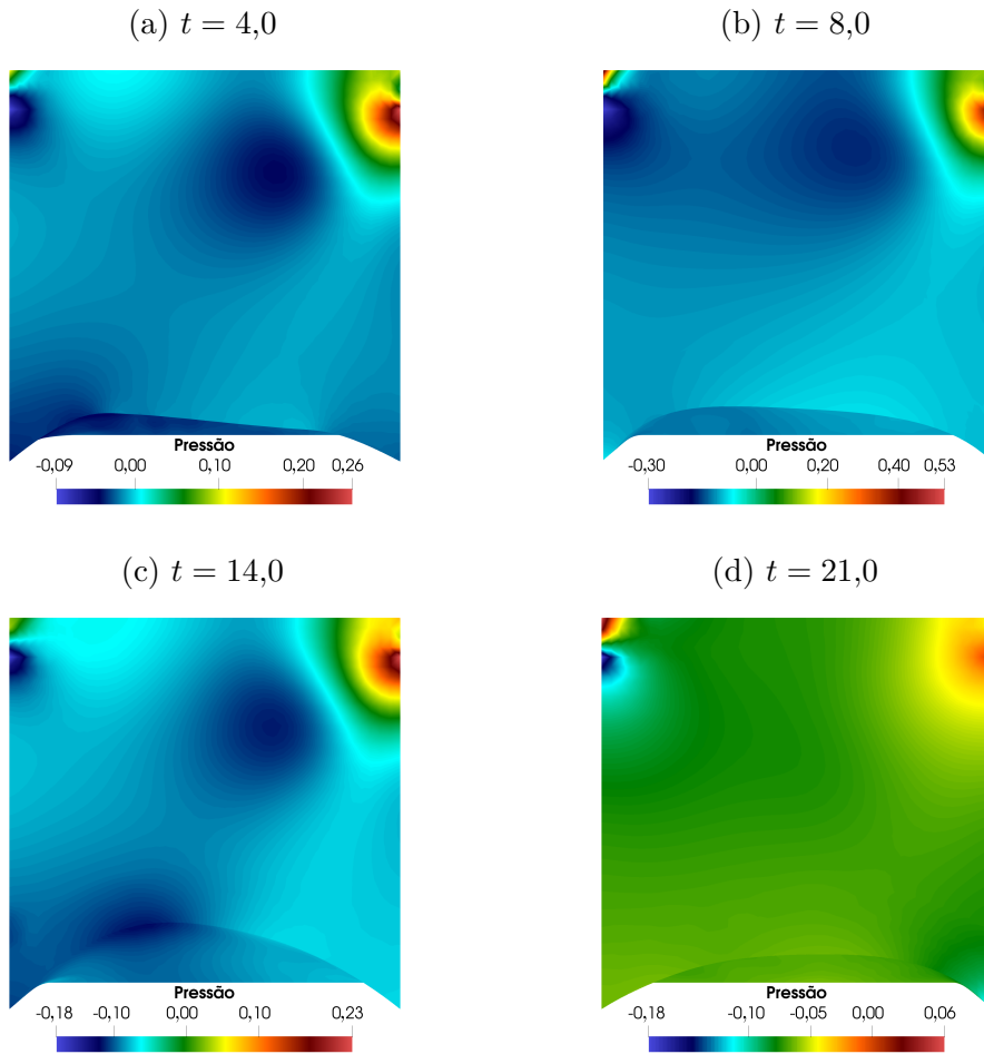
Figura 84 – Cavidade com fundo flexível 3D: campo de pressão
