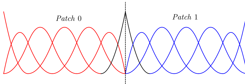
Figura 20 – Funções-base na interface entre patches
