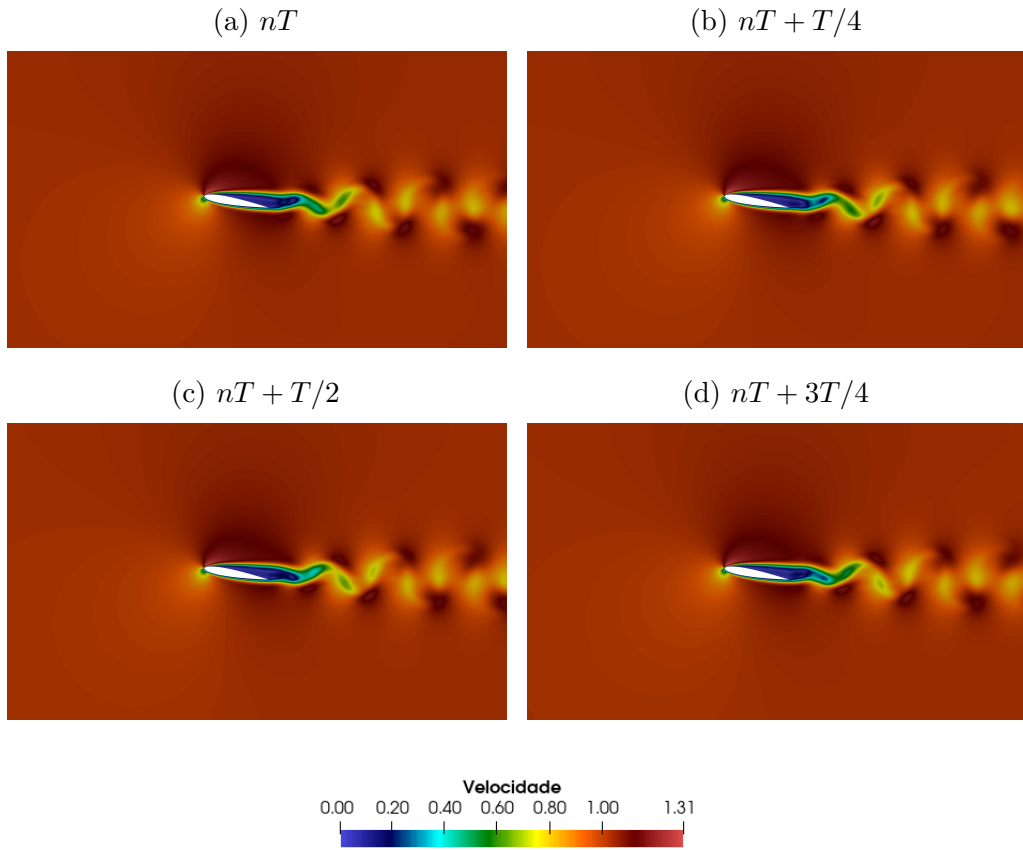
Figura 66 – Aerofólio: campo de velocidade
