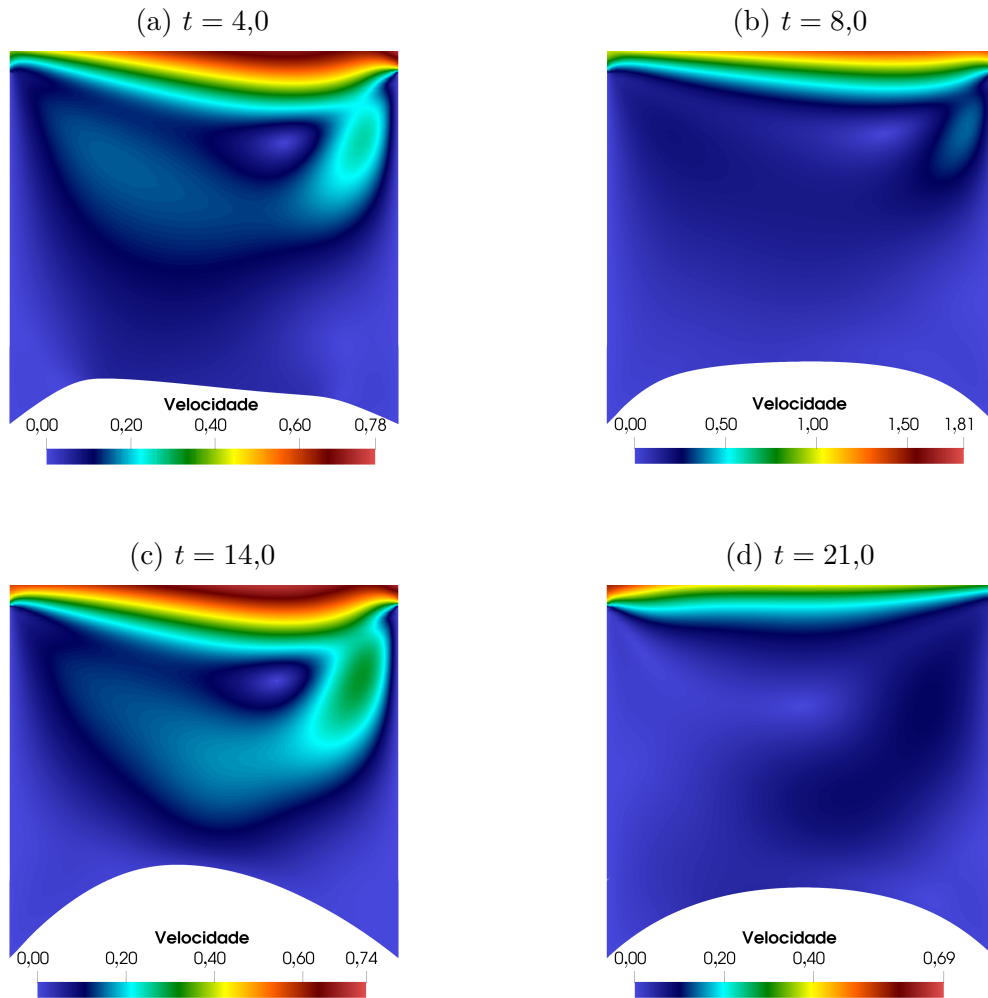
Figura 78 – Cavidade com fundo flexível 2D: campo de velocidade
