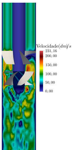
Figura 103 – Turbina modelo Arlequin: campo de velocidade
