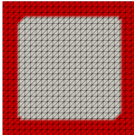
Figura 53 – Cavidade: nós desativados da malha global
