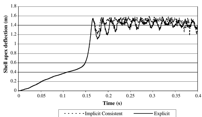
Figura 47 – Casca: deslocamento vertical nó central A - referência
