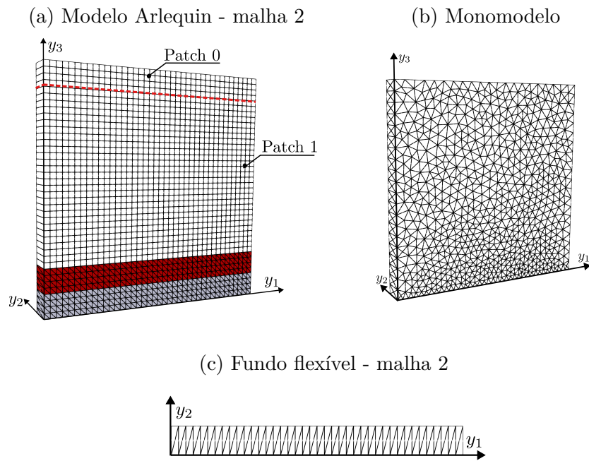
Figura 76 – Cavidade com fundo flexível 2D: discretizações
