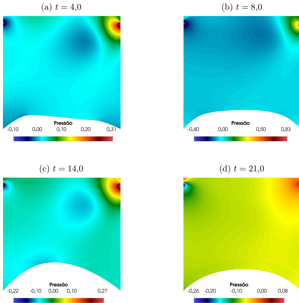
Figura 79 – Cavity com fundo flexível 2D: campo de pressão
