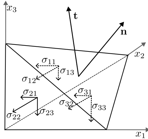
Figura 41 – Tetraedro elementar
