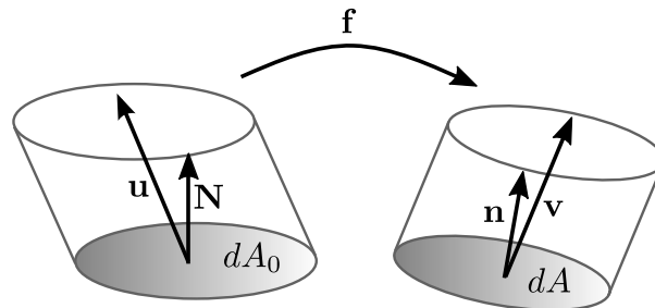
Figura 39 – Mudança de área
