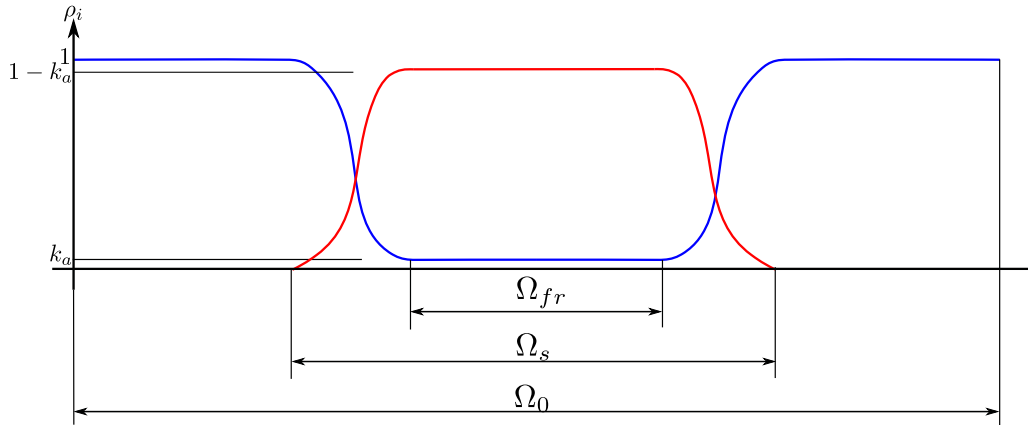
Figura 59 – Função ponderadora
