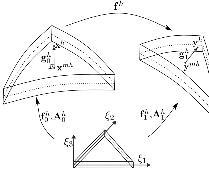
Figura 44 – Vetores generalizados
