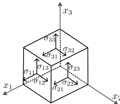
Figura 40 – Volume infinitesimal: componentes de tensão
