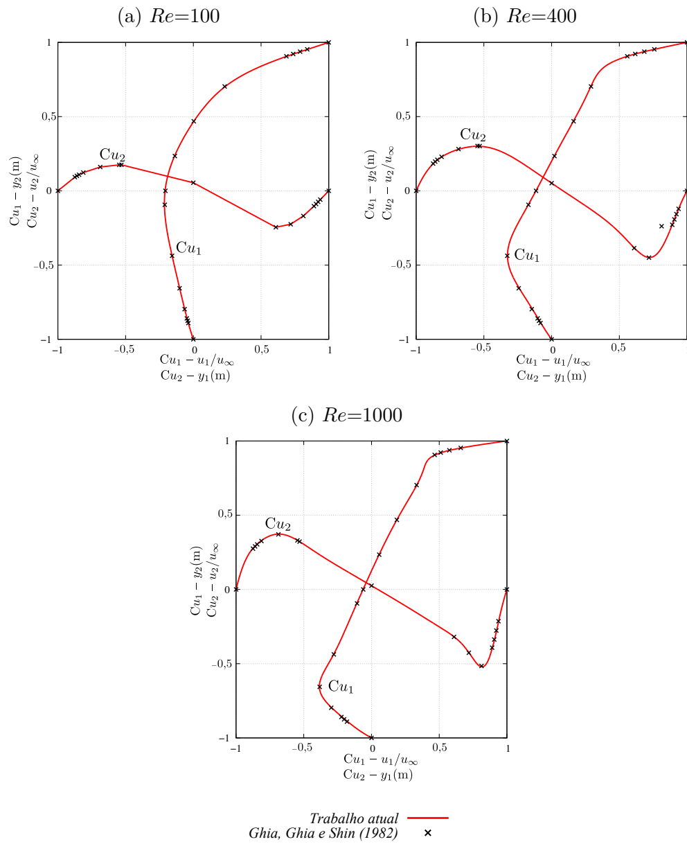
Figura 12 – Cavidade: perfis de velocidade adimensionalizados
