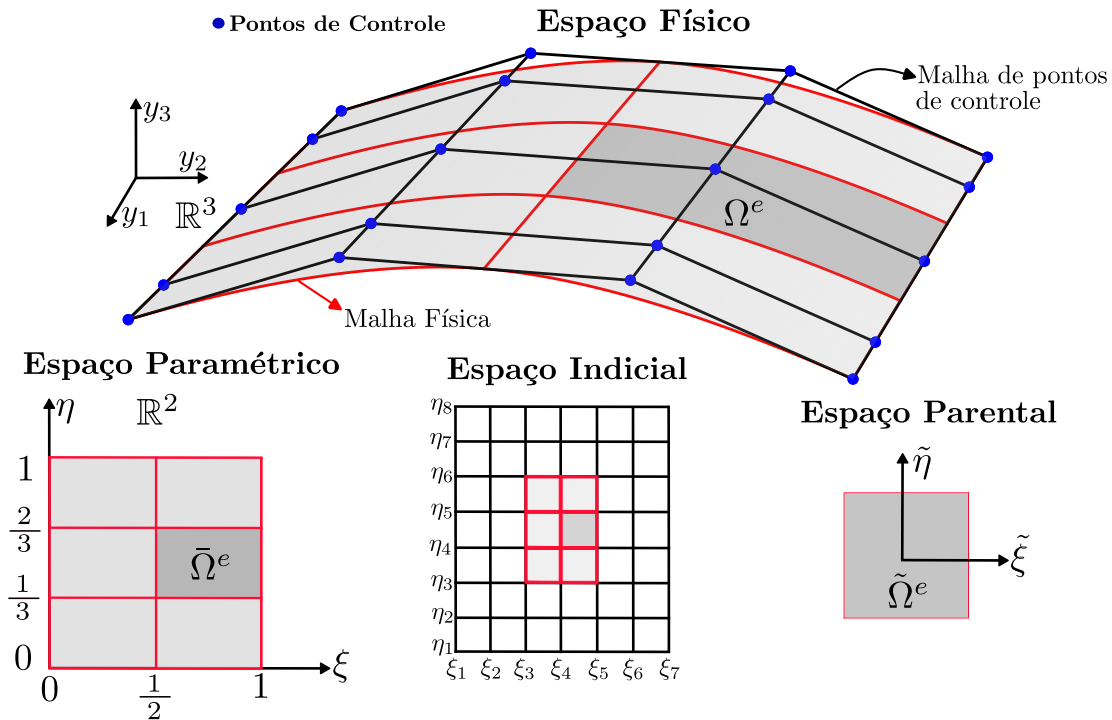
Figura 15 – NURBS: representação geométrica
