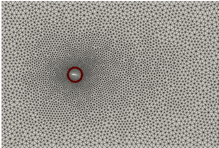
Figura 56 – Aerofólio: malhas global (MEF) e local (MEF)
