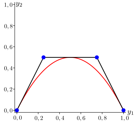
Figura 18 – Refinamento h de uma curva B -Spline
