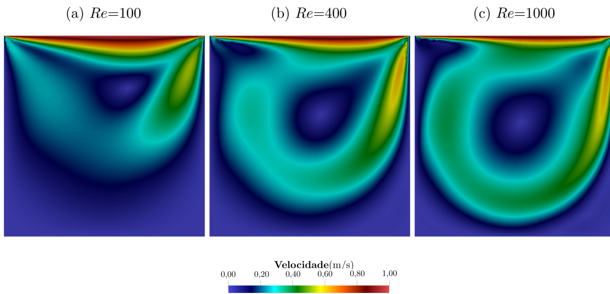
Figura 13 – Cavity: campo de velocidade
