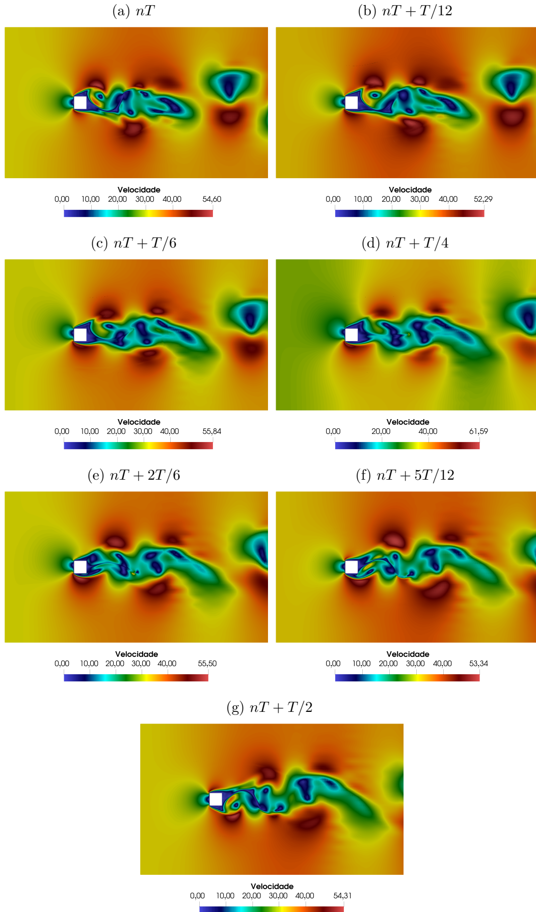
Figura 91 – Painel flexível: campo de velocidade
