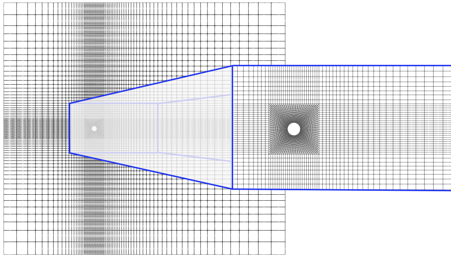
Figura 26 – Cilindro: malha de células físicas
