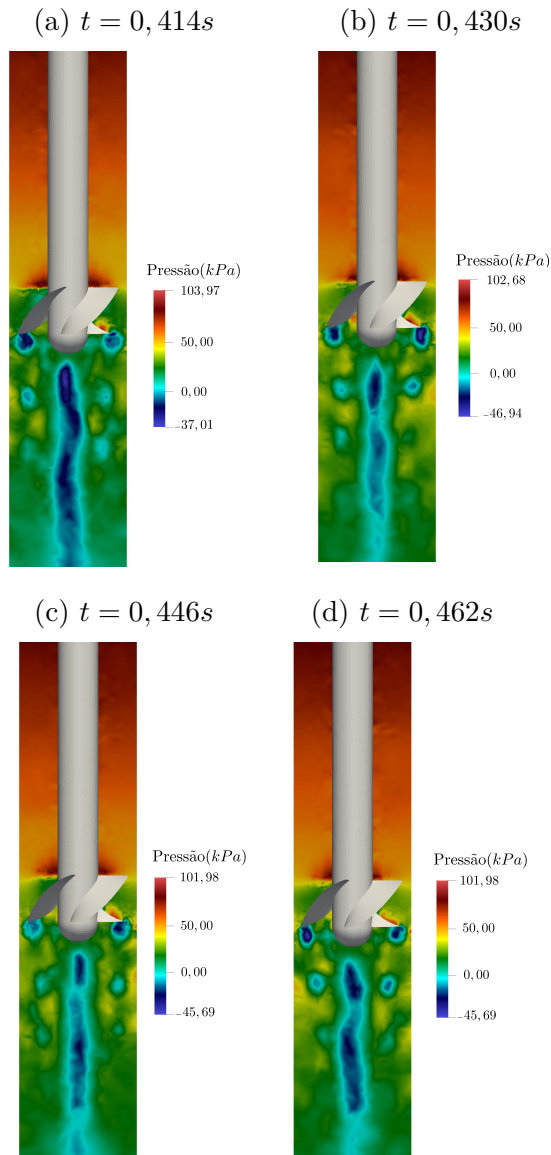
Figura 98 – Turbina monomodelo: campo de pressão
