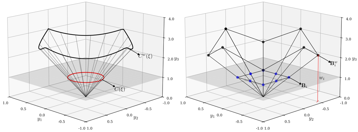
Figura 19 – Projeção transformativa de entidade B-Spline
