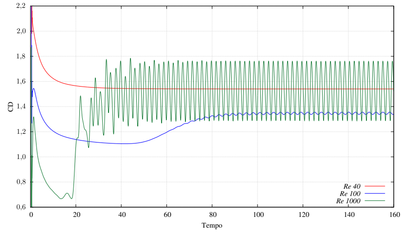
Figura 8 – Cilindro: coeficientes aerodinâmicos
