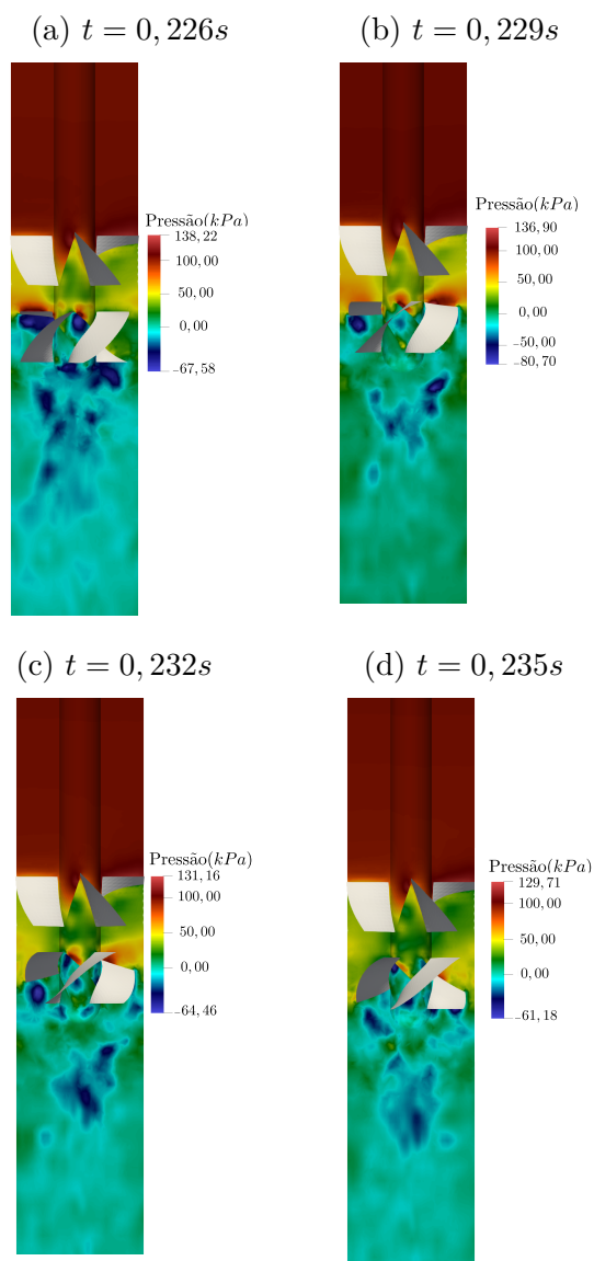
Figura 104 – Turbina modelo Arlequin: campo de pressão
