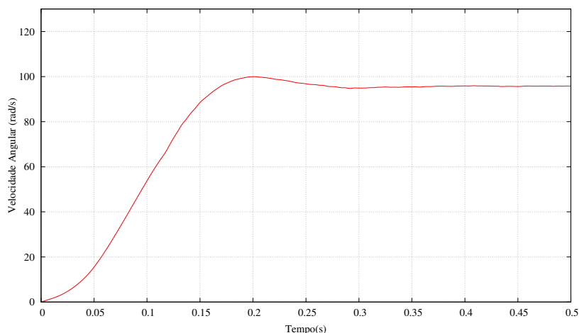
Figura 96 – Turbina monomodelo: velocidade angular no ponto A
