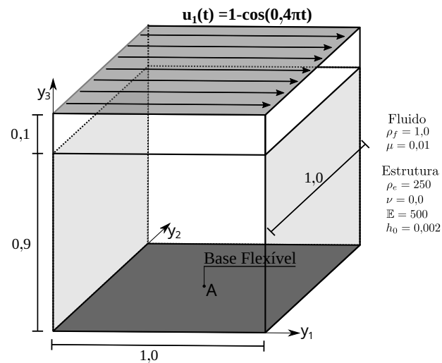
Figura 80 – Cavity com fundo flexível 3D: geometria e propriedades físicas
