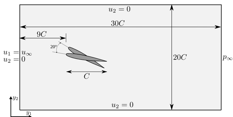
Figura 68 – Aerofólio Mov.: geometria
