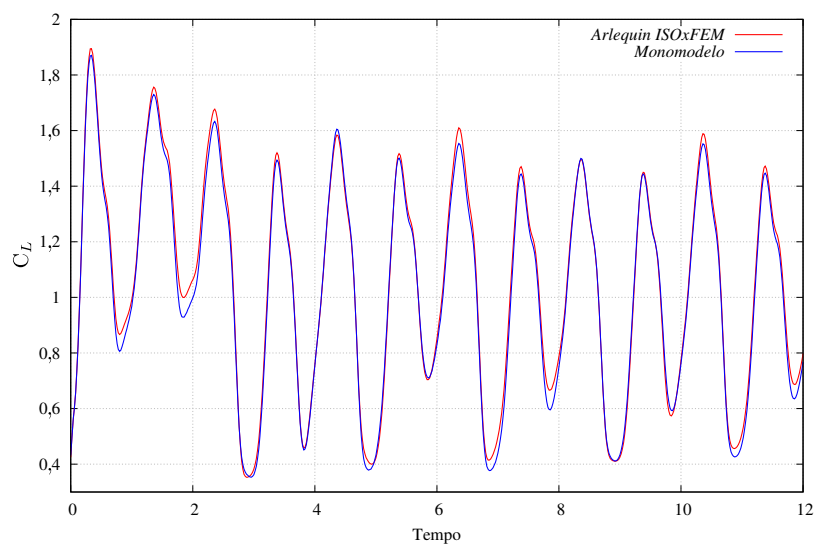
Figura 70 – Aerofólio Mov.: coeficiente de sustentação
