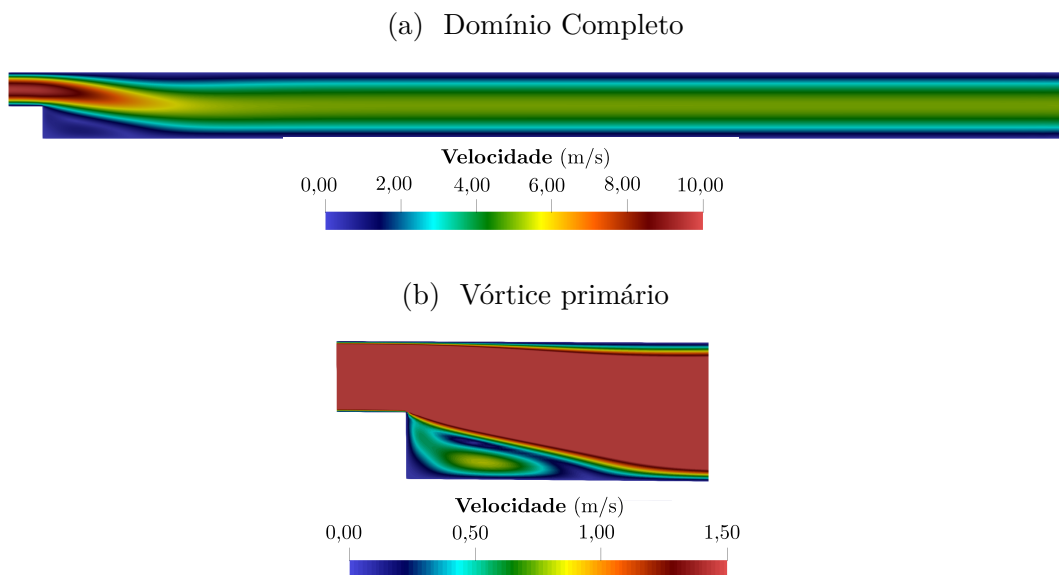
Figura 33 – Degrau: campo de velocidade para Re = 100
