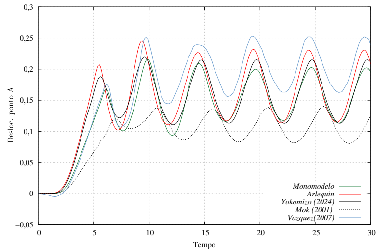
Figura 82 – Cavity com fundo flexível 3D: deslocamento do ponto A
