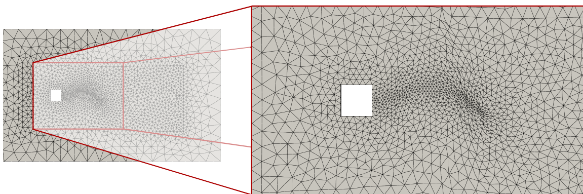
Figura 88 – Painel flexível: colapso malha monomodelo
