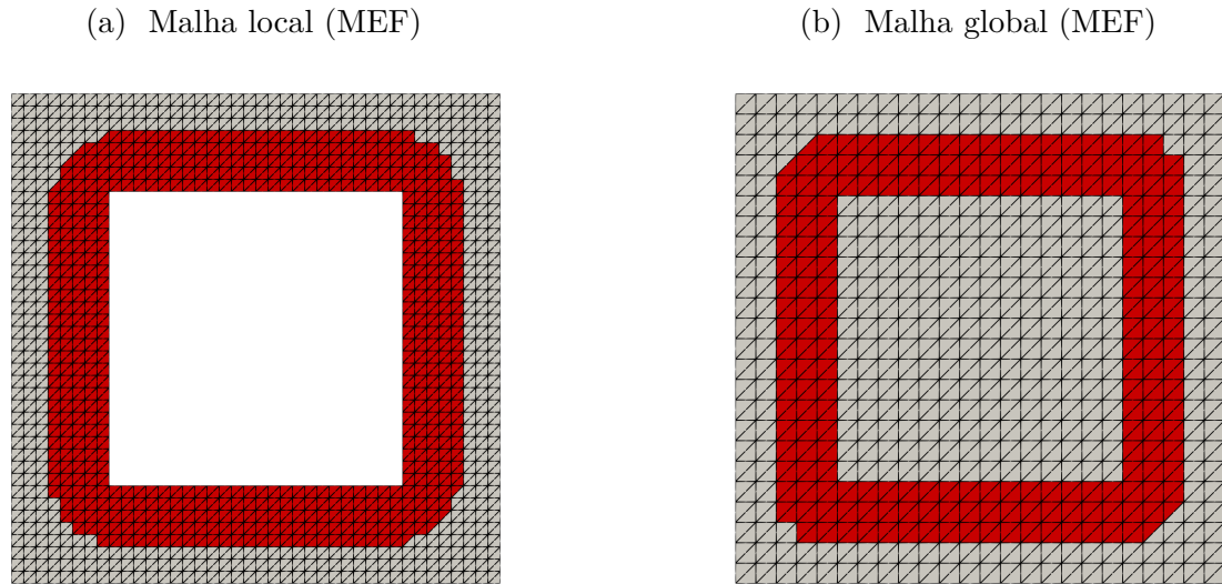
Figura 52 – Cavidade: malhas global e local
