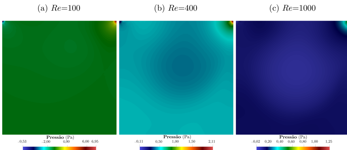
Figura 14 – Cavity: campo de pressão
