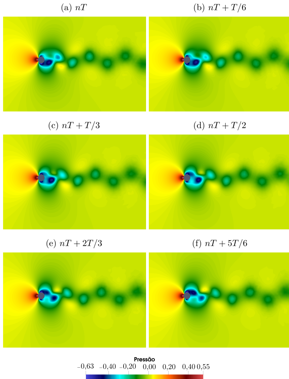
Figura 10 – Cilindro: campo de pressão para Re = 100
