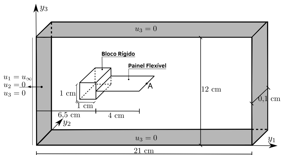
Figura 86 – Painel flexível: geometria e condições de contorno
