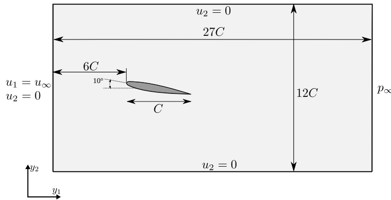
Figura 61 – Aerofólio: geometria
