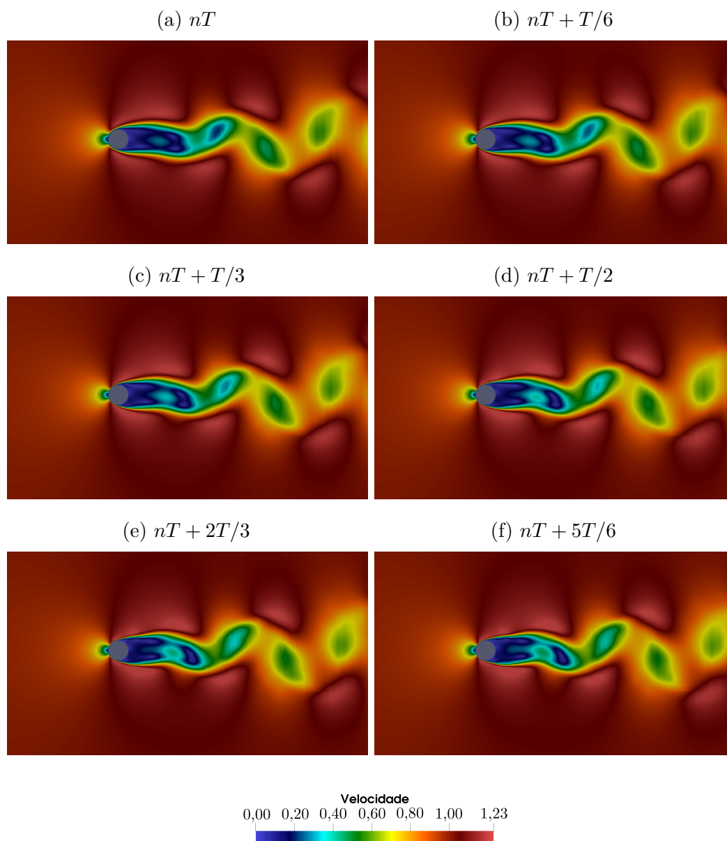
Figura 28 – Cilindro: campo de velocidade para Re = 1000
