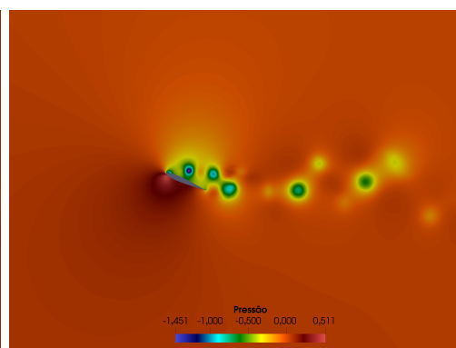
Figura 72 – Aerofólio Mov.: campo de pressão
