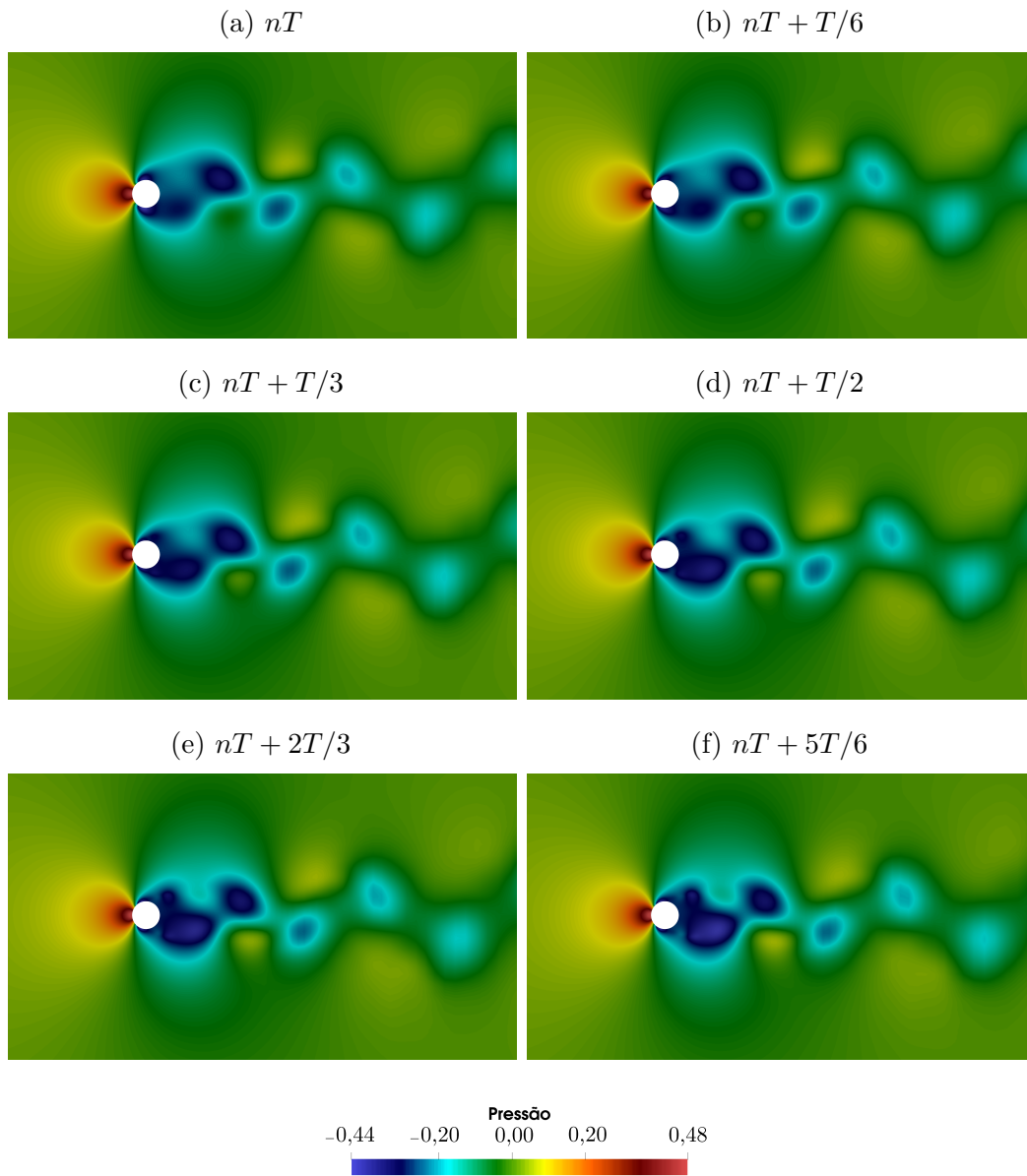
Figura 29 – Cilindro: campo de pressão para Re = 1000
