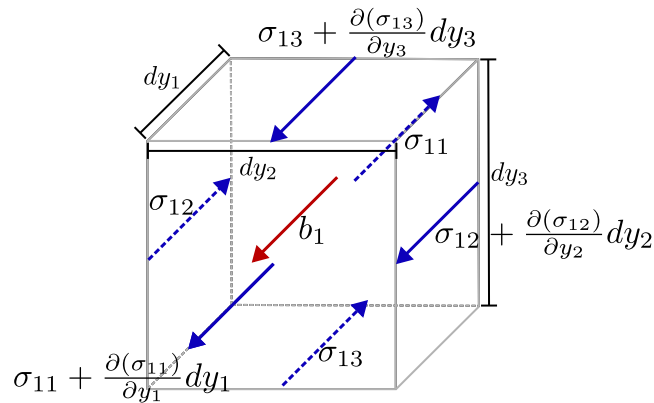
Figura 2 – Volume de controle infinitesimal: componentes de força na direção y_1
