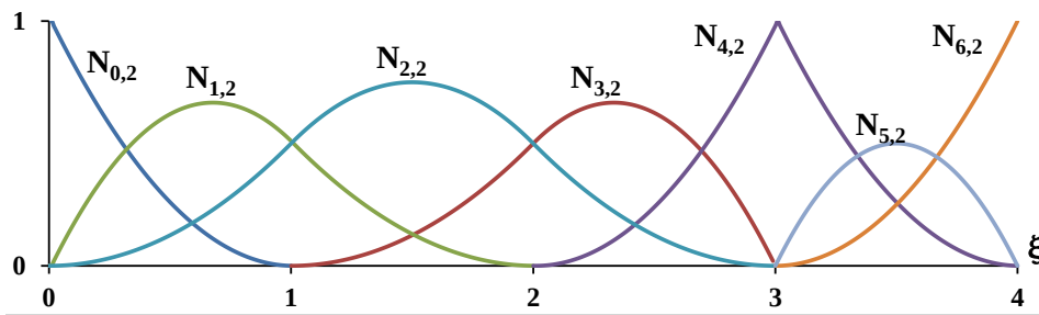
Figura 16 – Funções B-Splines
