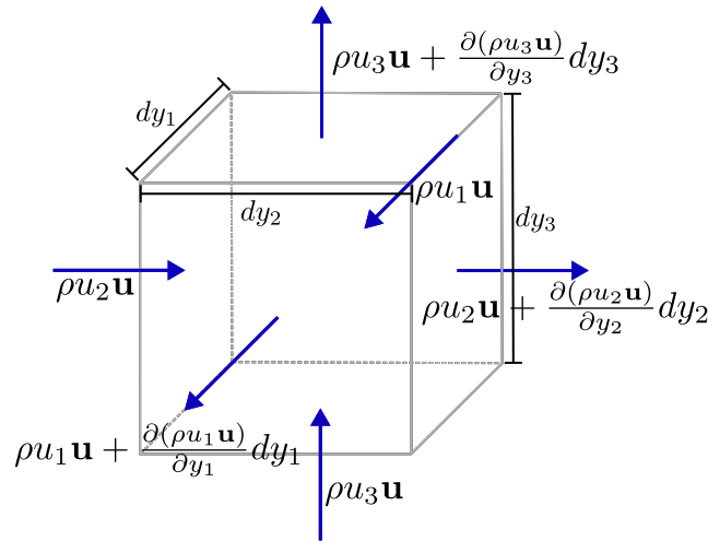
Figura 3 – Volume de controle infinitesimal: fluxo de quantidade de movimento
