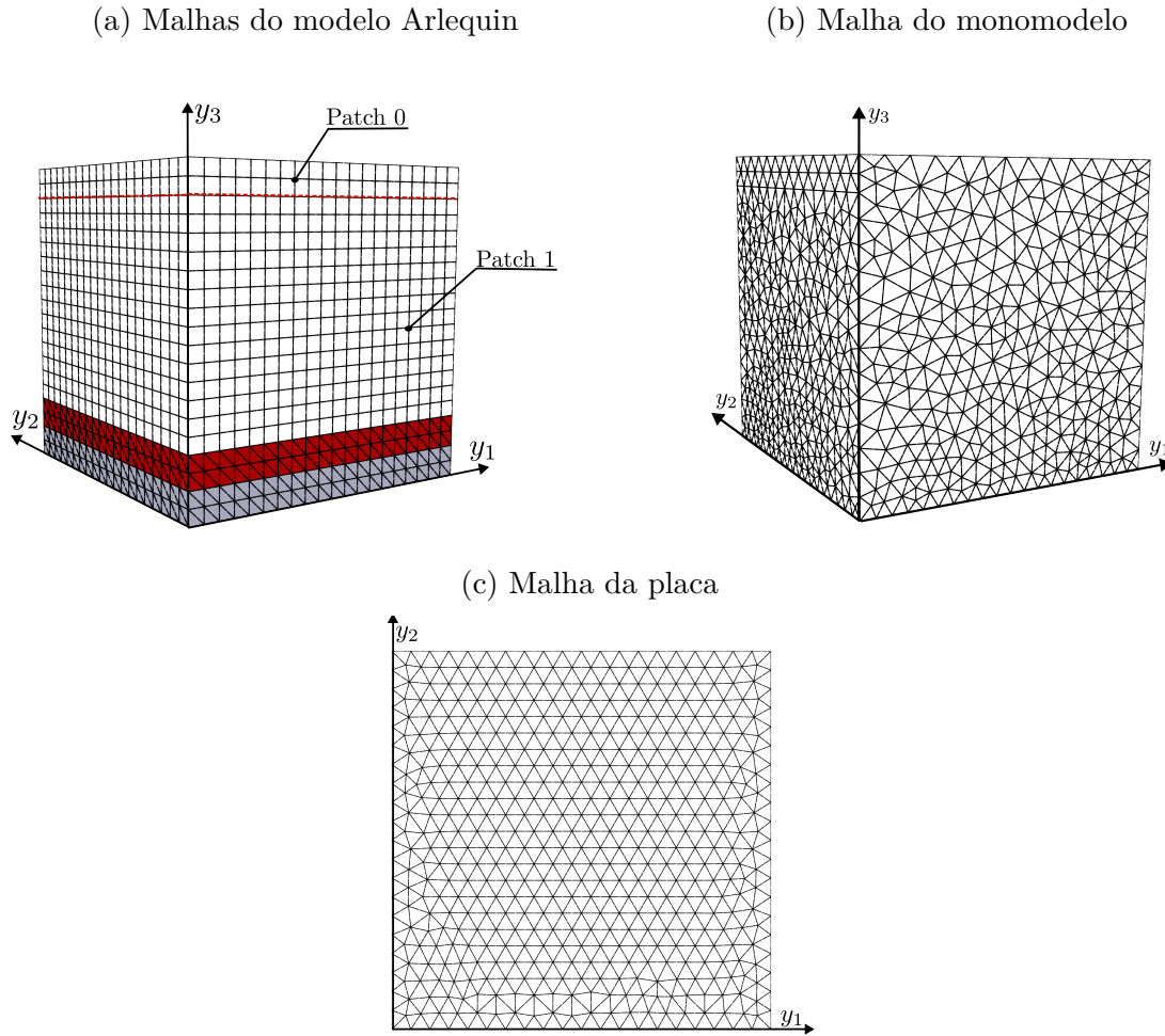
Figura 81 – Cavidade com fundo flexível 3D: discretização
