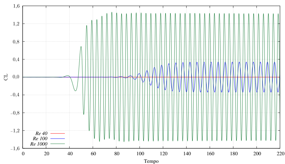
(b) Coeficiente de sustentação C_L
