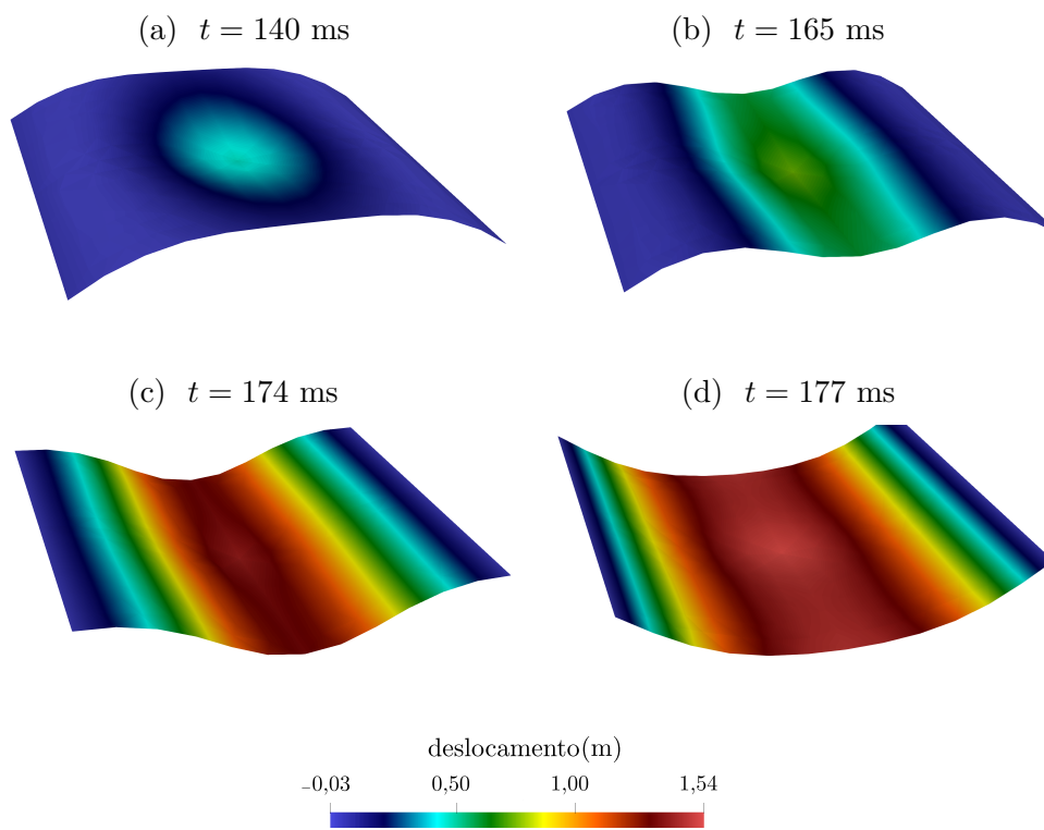
Figura 48 – Casca: campo de deslocamento
