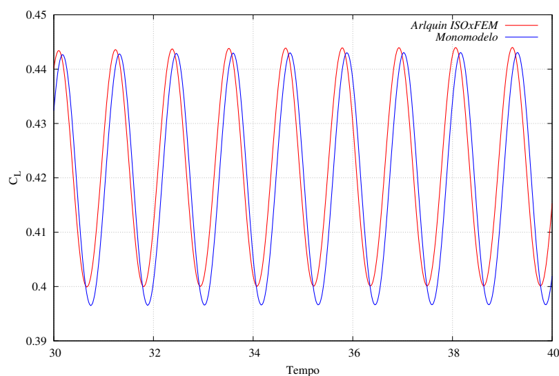
Figura 65 – Aerofólio: coeficiente de sustentação
