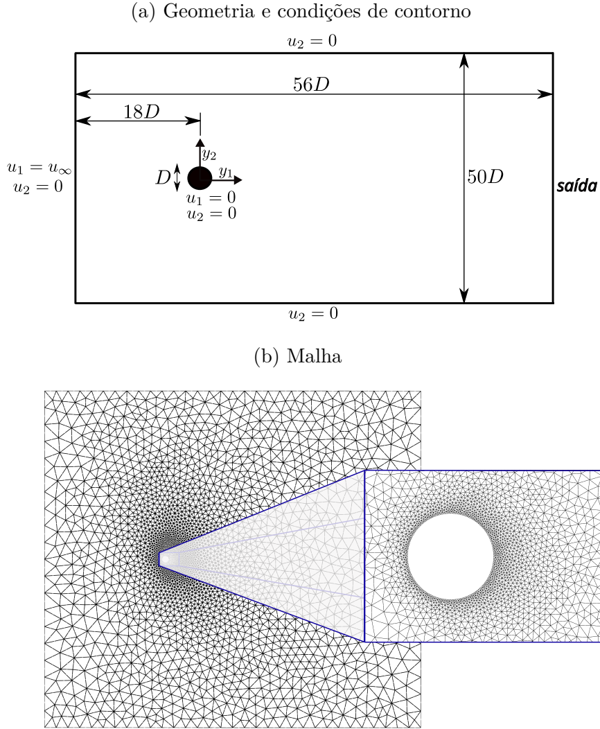
Figura 7 – Cilindro: geometria, condições de contorno e malha
