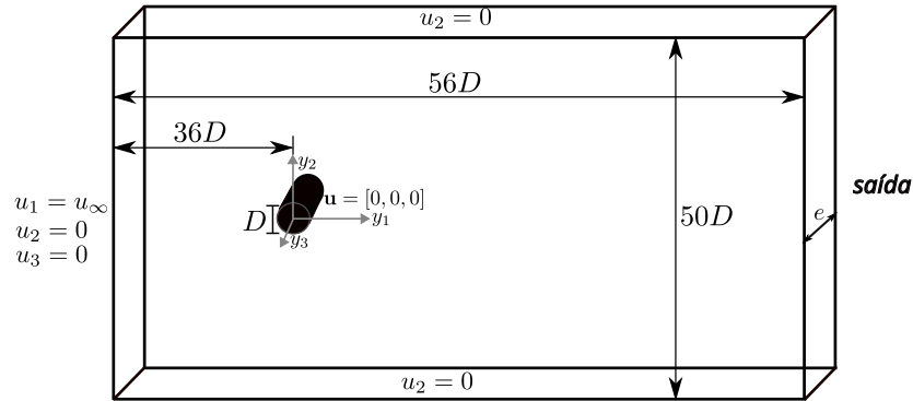
Figura 21 – Cilindro: geometria e condições de contorno
