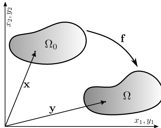
Figura 37 – Cinemática de um sólido deformável
