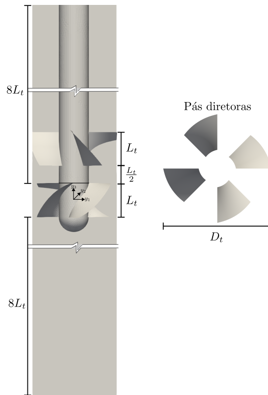
Figura 99 – Turbina modelo Arlequin: geometria
