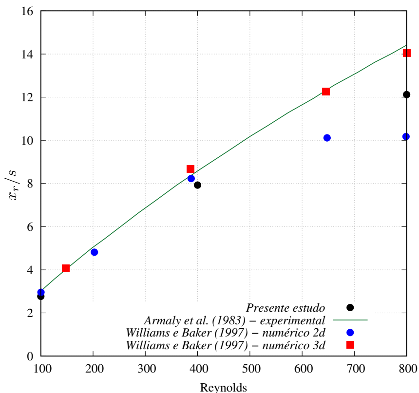
Figura 32 – Degrau: comprimento do vórtice principal
