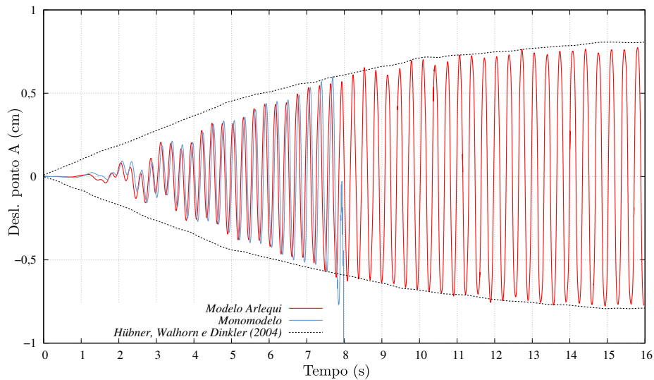
Figura 89 – Painel flexível: deslocamento em A
