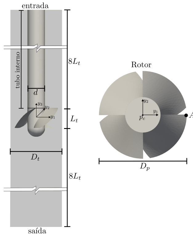
Figura 93 – Turbina monomodelo: geometria
