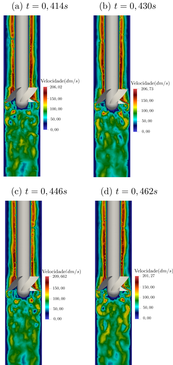
Figura 97 – Turbina monomodelo: campo de velocidade
