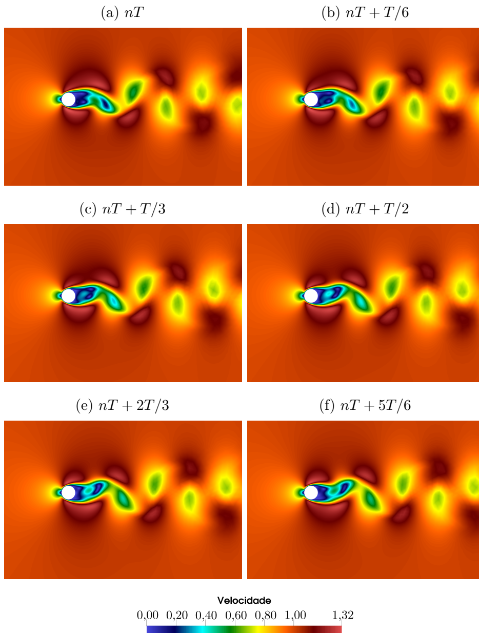
Figura 9 – Cilindro: campo de velocidade para Re = 100
