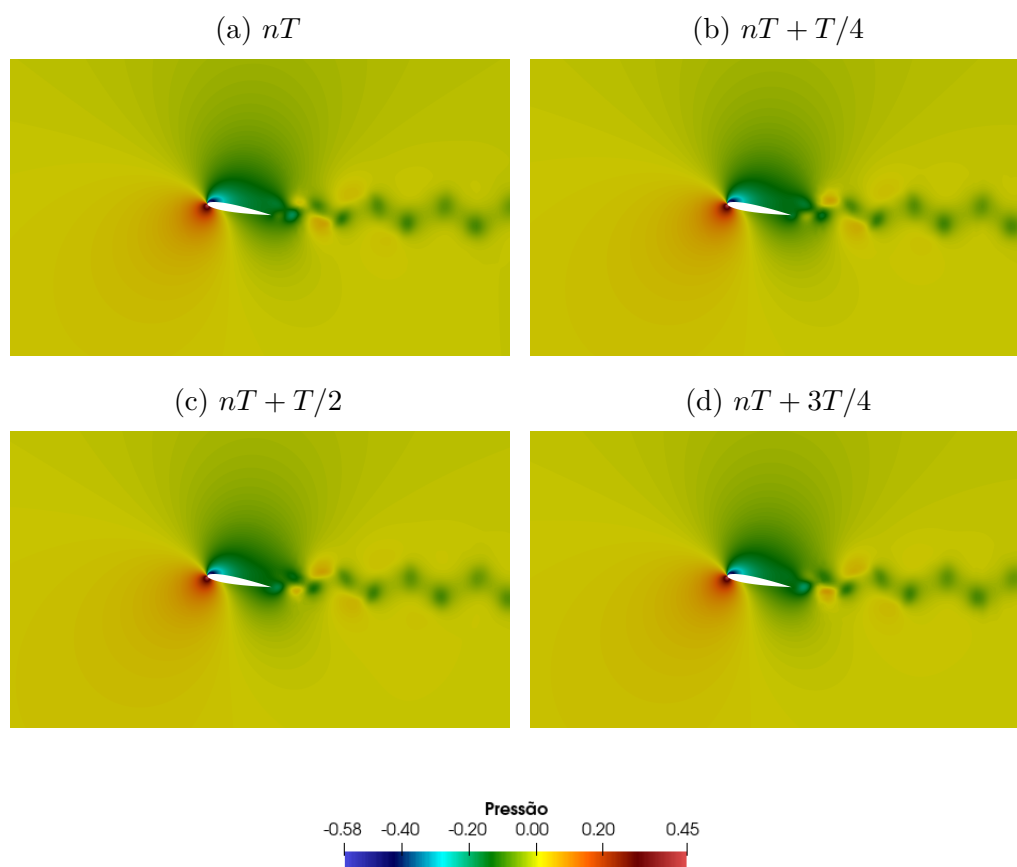
Figura 67 – Aerofólio: campo de pressão
