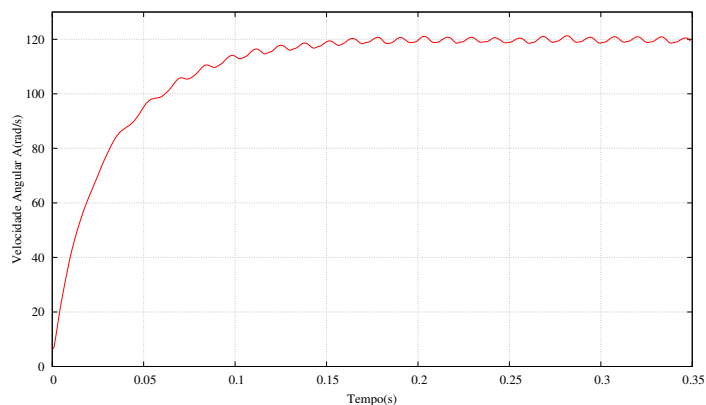
Figura 102 – Turbina modelo Arlequin: velocidade angular no ponto A
