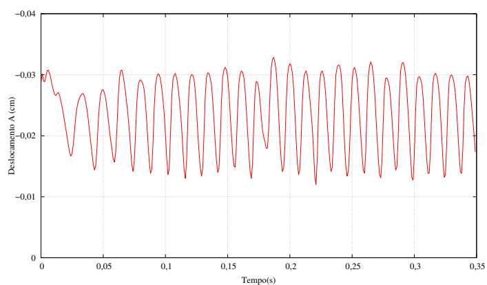
Figura 101 – Turbina modelo Arlequin: deslocamento no ponto A
