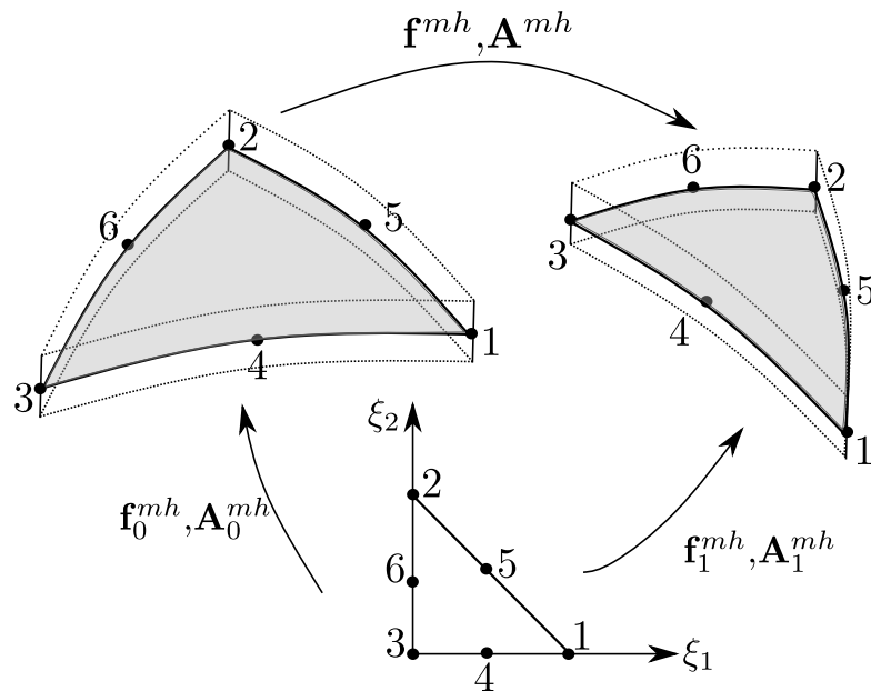
Figura 43 – Mapeamento da superfície média da casca
