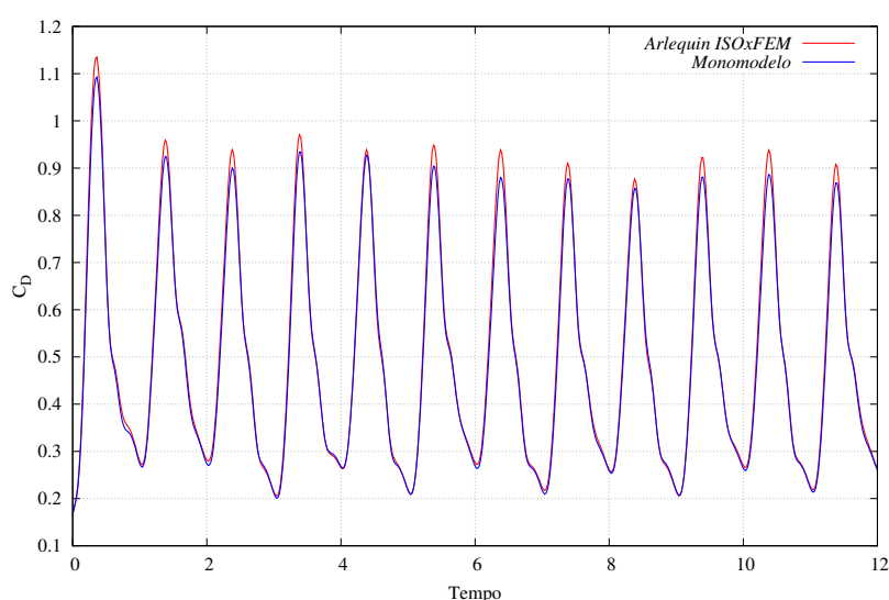
Figura 69 – Aerofólio Mov.: coeficiente de arrasto
