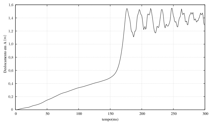
Figura 46 – Casca: deslocamento vertical nó central A
