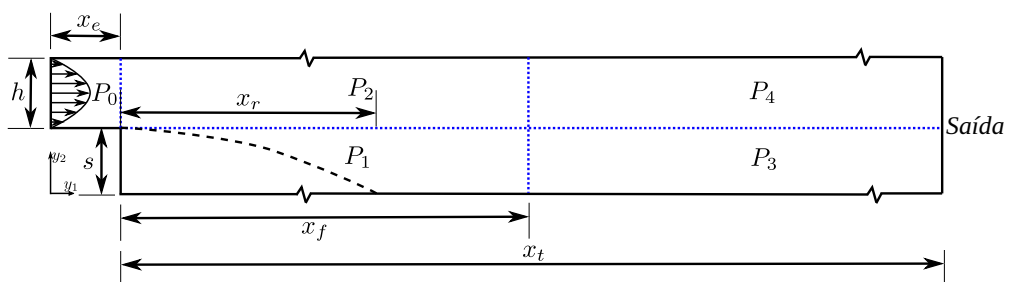
Figura 30 – Degrau: geometria
