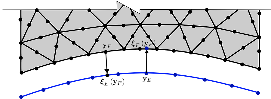
Figura 74 – Discretizações não-coincidentes no contorno de IFE
