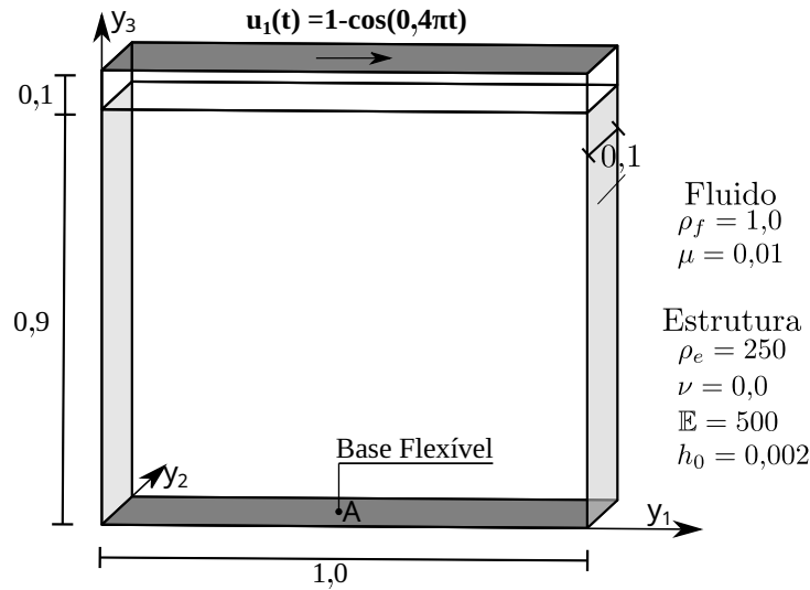
Figura 75 – Cavidade com fundo flexível 2D: geometria e propriedades físicas
