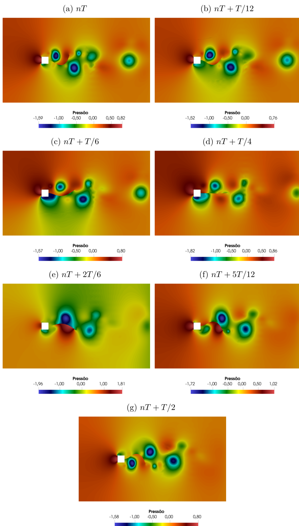
Figura 92 – Painel flexível: campo de pressão
